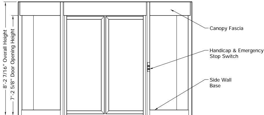
① Elevation
